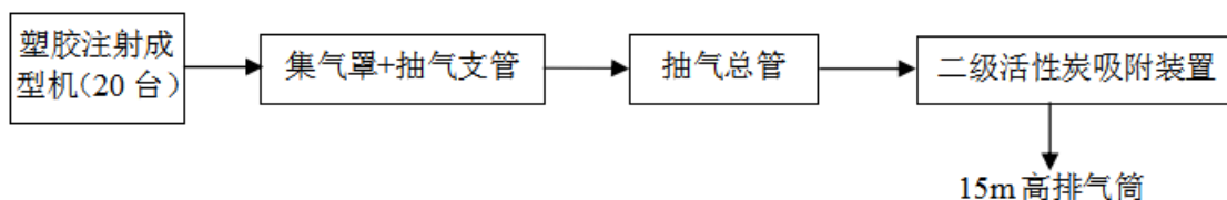
图 2.2-1 本项目塑料筐生产过程非甲烷总烃治理流程示意图
