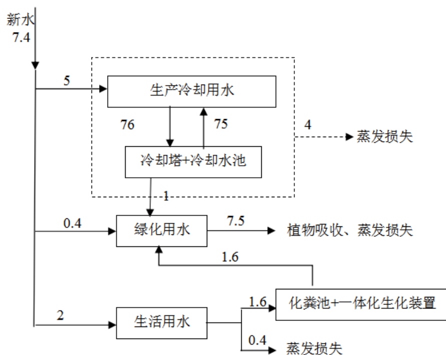
图 2.1-5 项目总水平衡图 (t/d)
